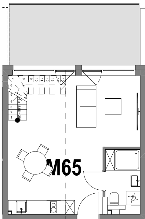
RZUT POZIOM +3
