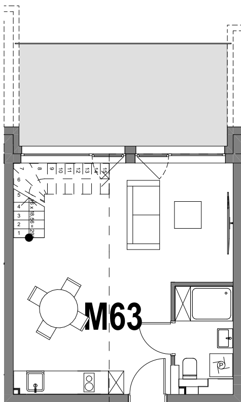
RZUT POZIOM +3
