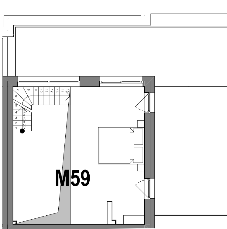
RZUT POZIOM ANTRESOLI
